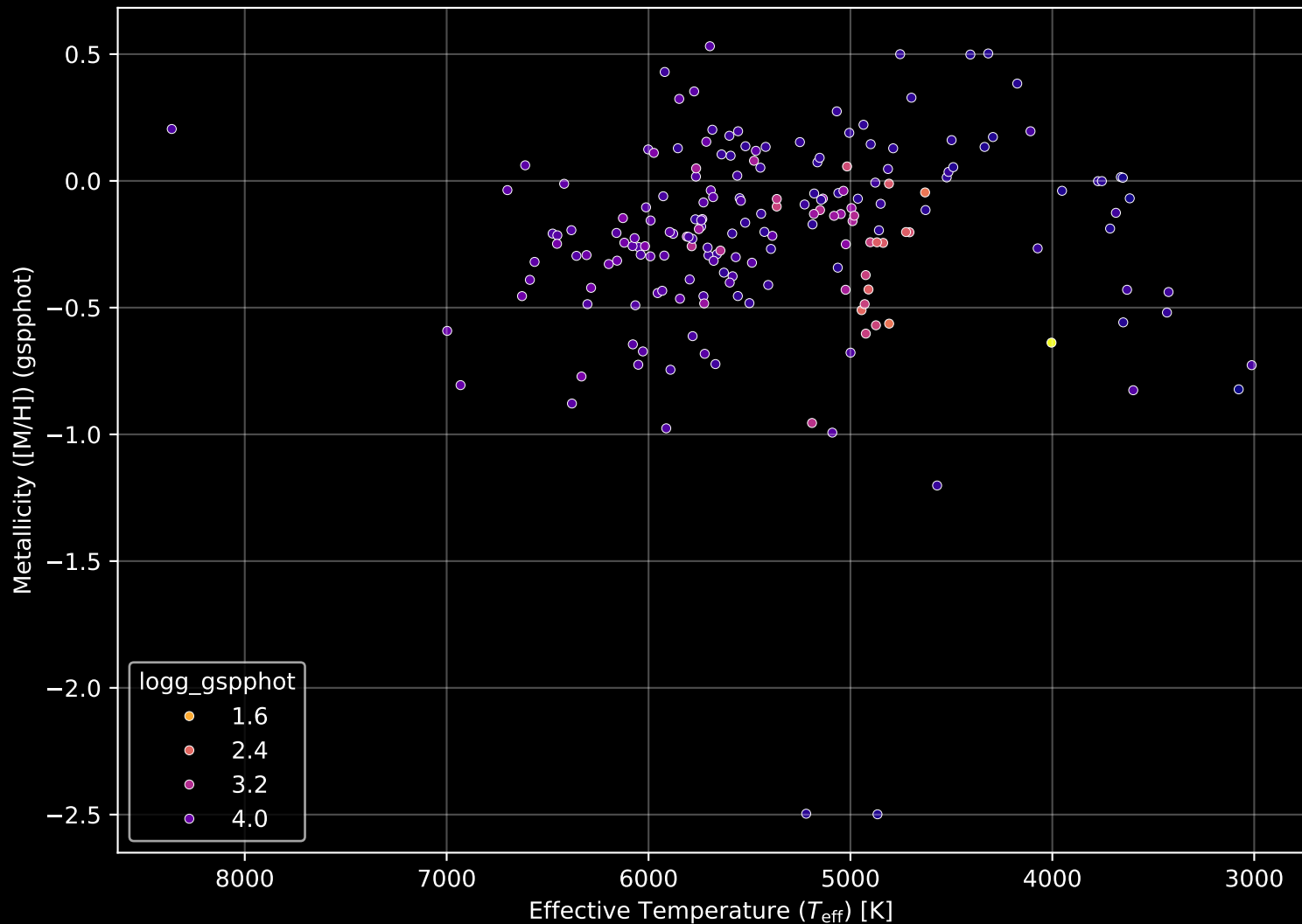
APOGEE DR17 Field: [102+61_MGA] Stellar Population Parameters (n= 188)
